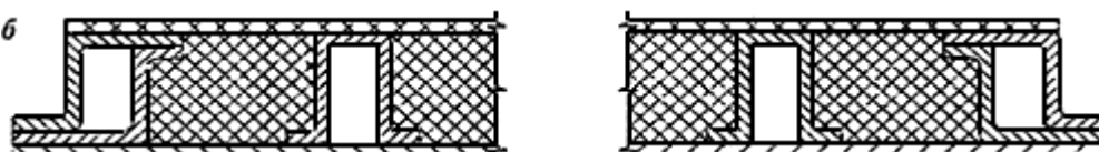
Полотно с наружным стальным листом и внутренним листом из ДВП, с профилями сложного сечения и наполнением из древесного или минерального утеплителя
